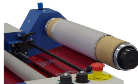
Dokončovací aplikátor (Foiler)
